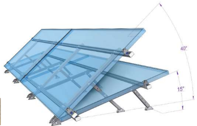
Elevación variable 15° a 40 °
